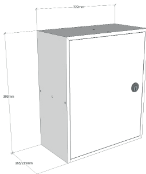
ONDERDEEL DEUR
